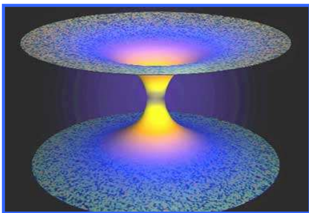
Antes del Big Bang: Colapso y expansión de universos indefinidamente
