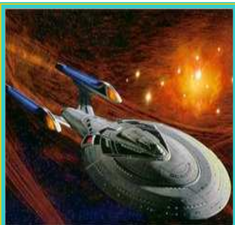
La serie de TV Star Trek, basada en el Multiverso
