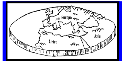
Tierra plana en la Edad media
