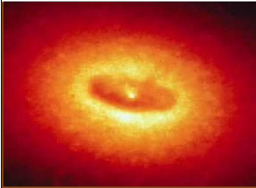
Gas y polvo alrededor de un agujero negro
