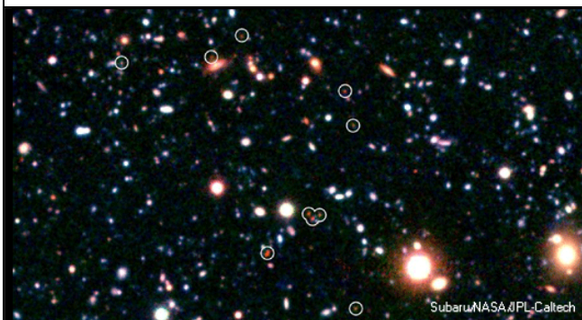
El cúmulo de galaxias más lejano, a 12.600 millones años luz
