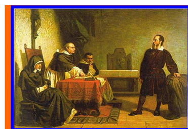
Proceso de Galileo
