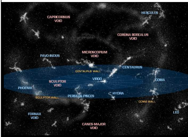
Supercúmulo de Virgo 200 millones años luz de diámetro
