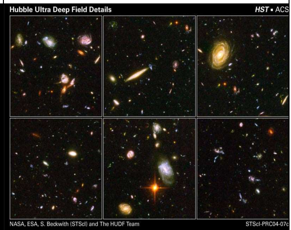
Galaxias a 5000 - 10000 millones años luz. Foto del telescopio Hubble
