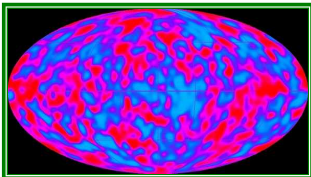
Diferentes temperaturas en la radiación de fondo detectadas por los satélites
