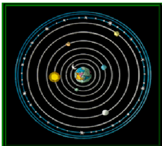
Modelo cosmológico de Ptolomeo con la Tierra en el centro
